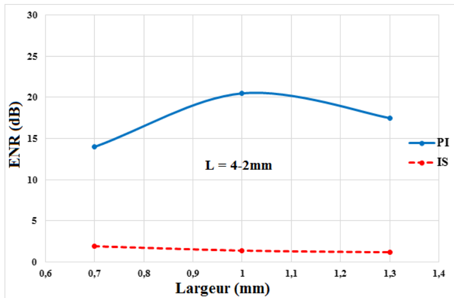
FIGURE III.15 – ENR en fonction de la largeur à 9,4GHz
