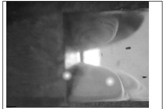
Figure 5 : Position diagonale des vortex à l'équilibre (contraction carré/carré) à \dot{\gamma}_a = 60 \text{ s}^{-1}
